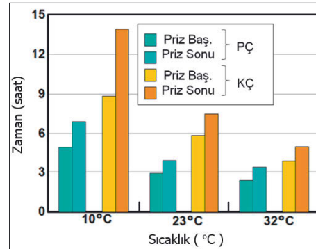
Şekil 8: Beton sıcaklığı-priz süresi ilişkisi [6]
