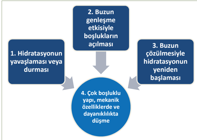
Şekil 3: Donma-çözülmenin taze betona etkisi
